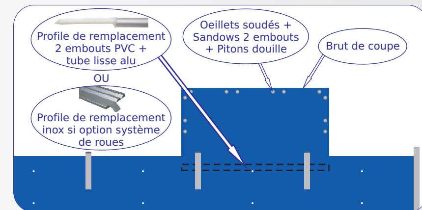
ESCALIER SUR LA LONGUEUR DE LA PISCINE
