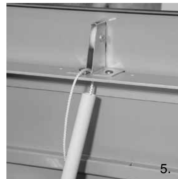
Skizze Schnurführung Section string guiding Dessin passage de la ficelle
