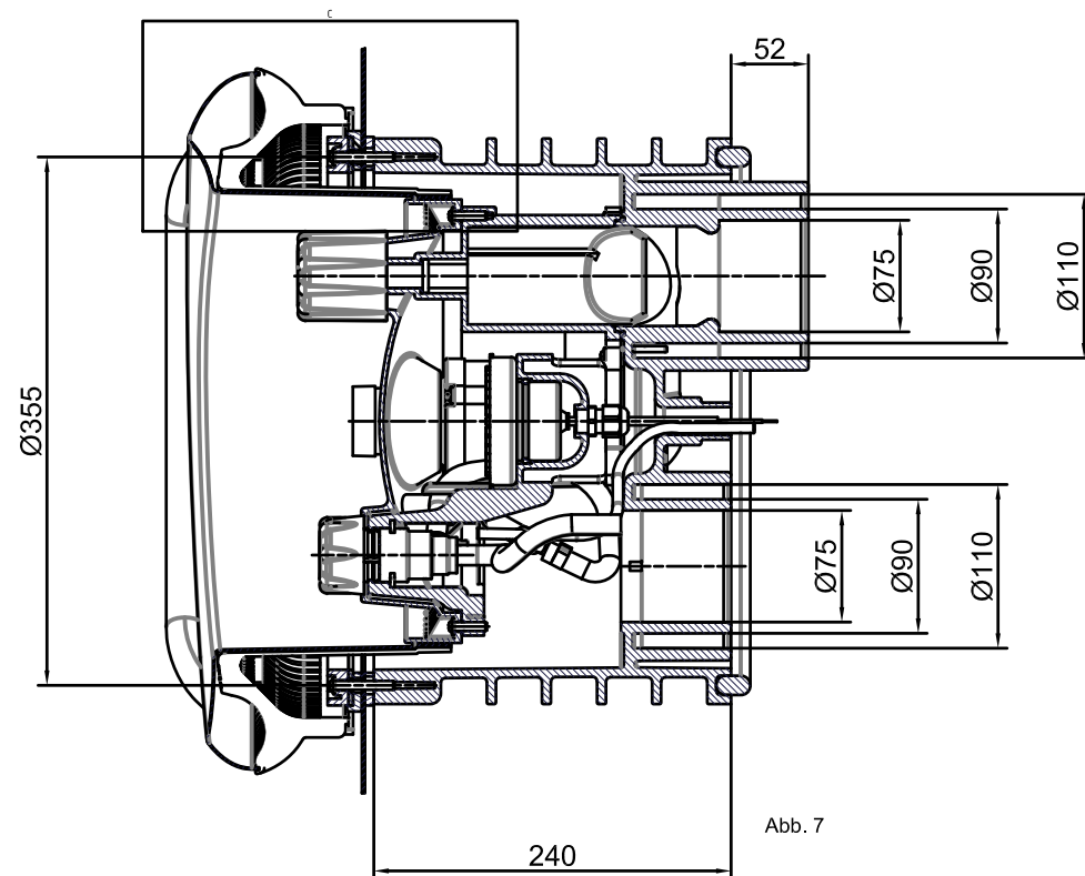
A-A ( 1 : 1 )
