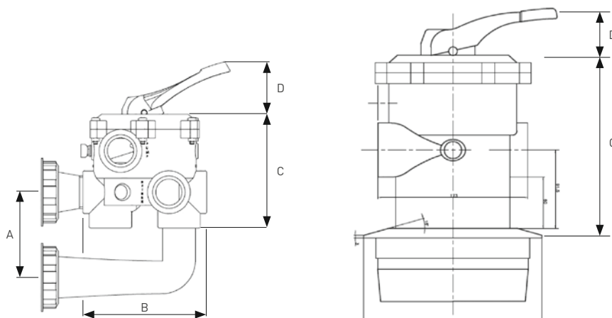
Válvula Lateral
